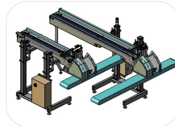
0.3 Clippy su linea di confezionamento/ Systems on a production line
